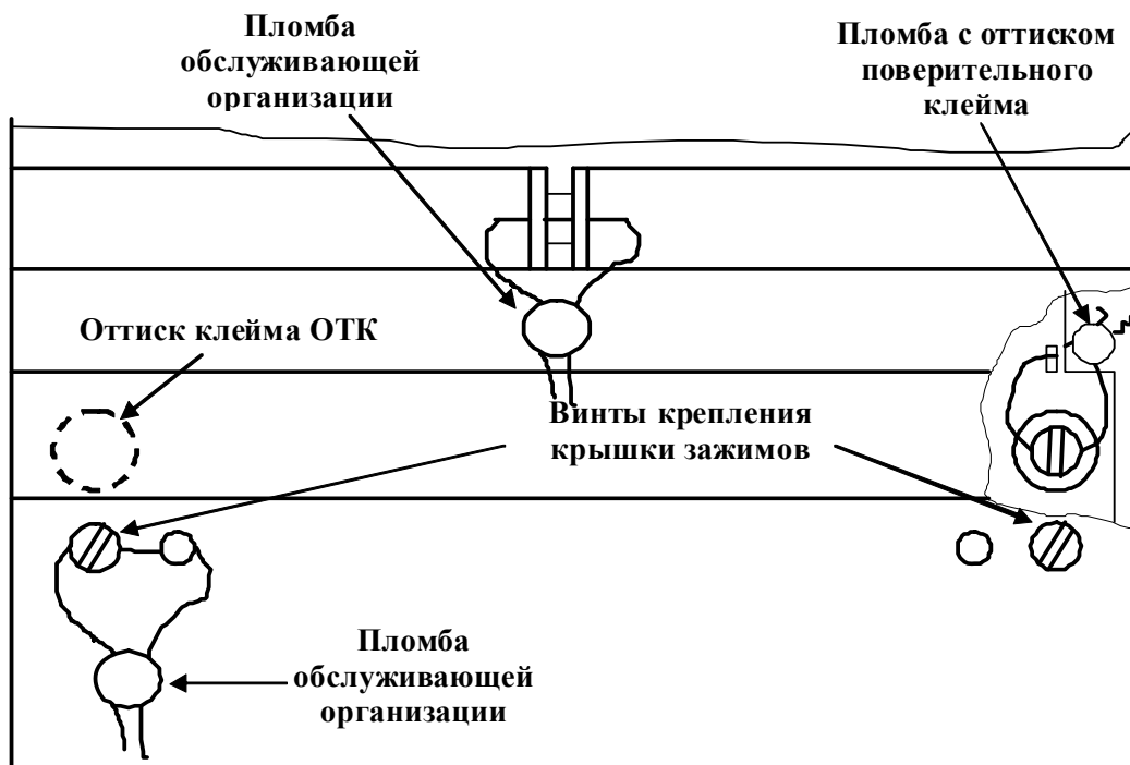
Рисунок 33 – Пломбирование счетчика и крепление крышки зажимов
