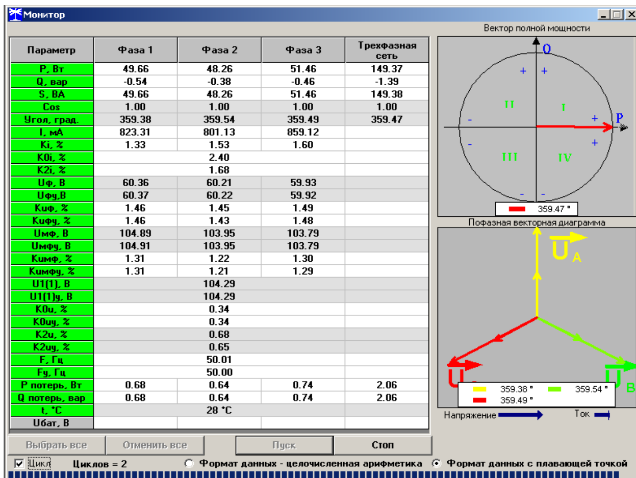
Рисунок 28 – Форма «Монитор»
