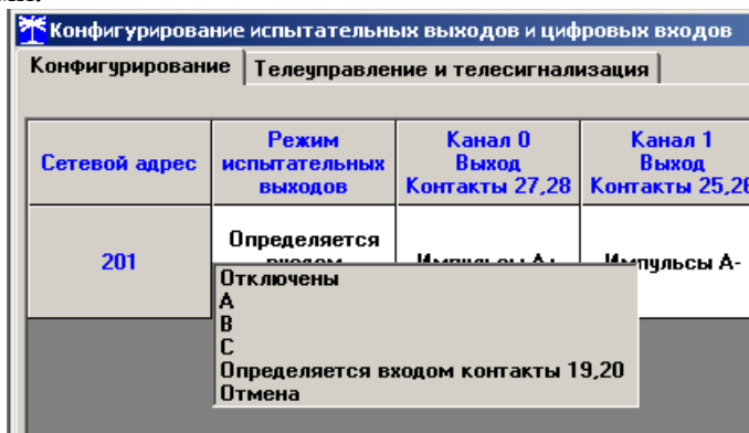
Рисунок 25 – Вкладка «Конфигурирование»
